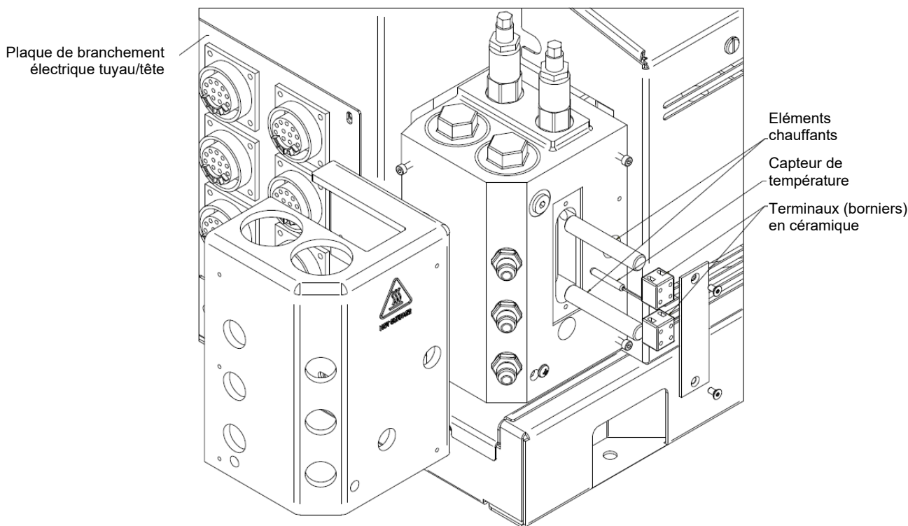
Collecteur de filtre à double sortie en option
