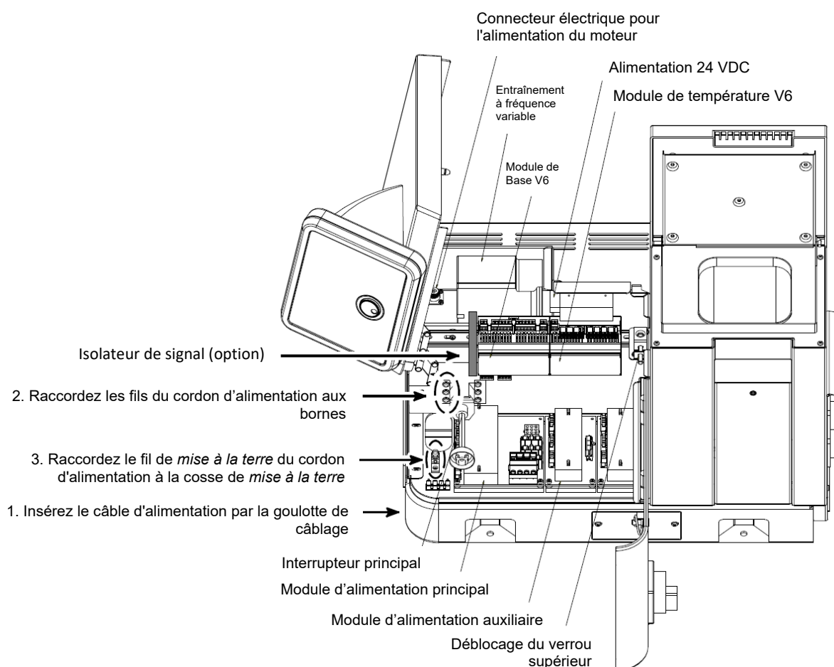
Montage de l'alimentation principale & les composants internes
