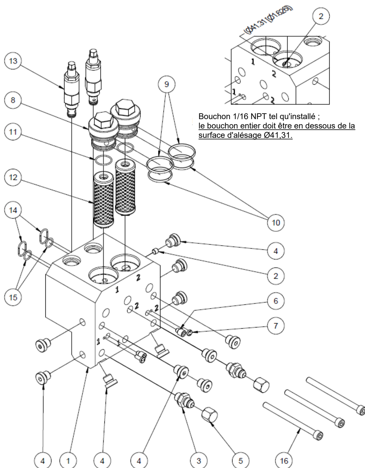
Illustration: Ensemble Collecteur de filtre à double sortie, DCL, SR22/45, NP 123441
