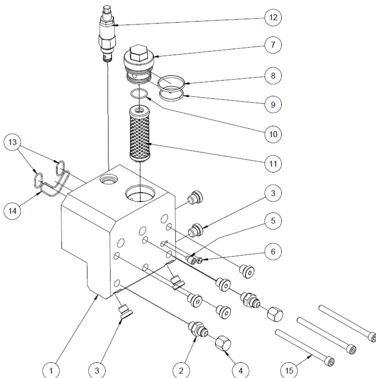
Illustration: Ensemble Collecteur de filtre à simple sortie, DCL, SR22/45, NP 123440
