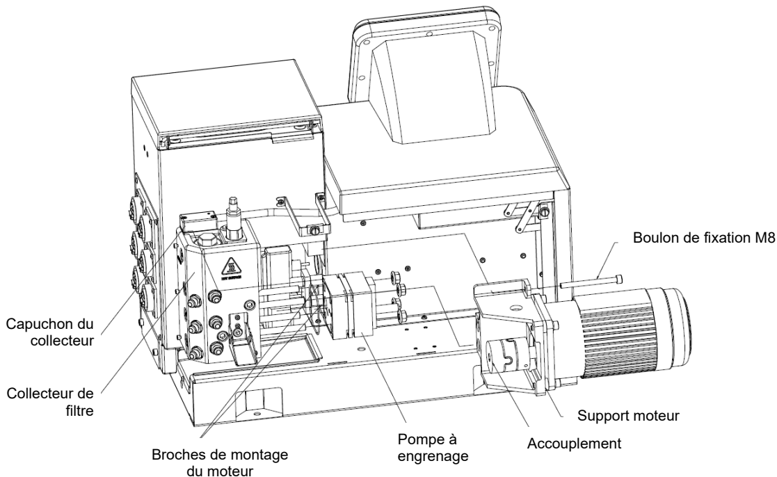
Modèle de pompe à engrenage avec collecteur de filtre à simple sortie, vue arrière
