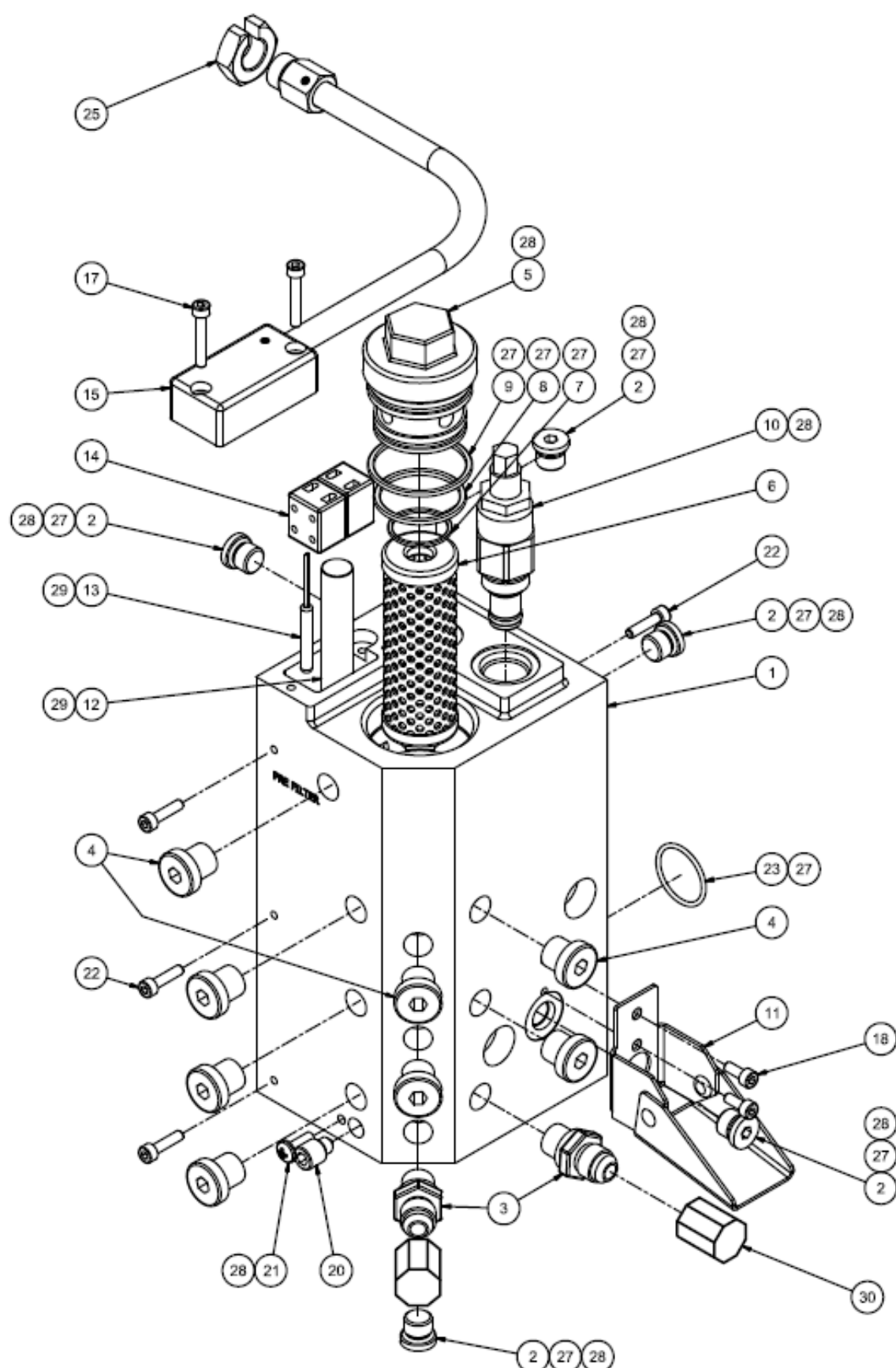
Illustration: Ensemble Collecteur de filtre à simple sortie, SR5/10
