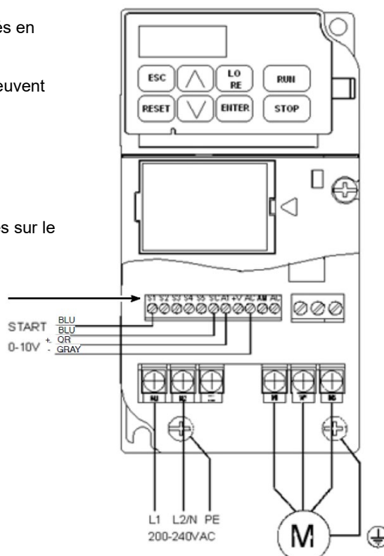
Disposition de l'entraînement de la commande du moteur
