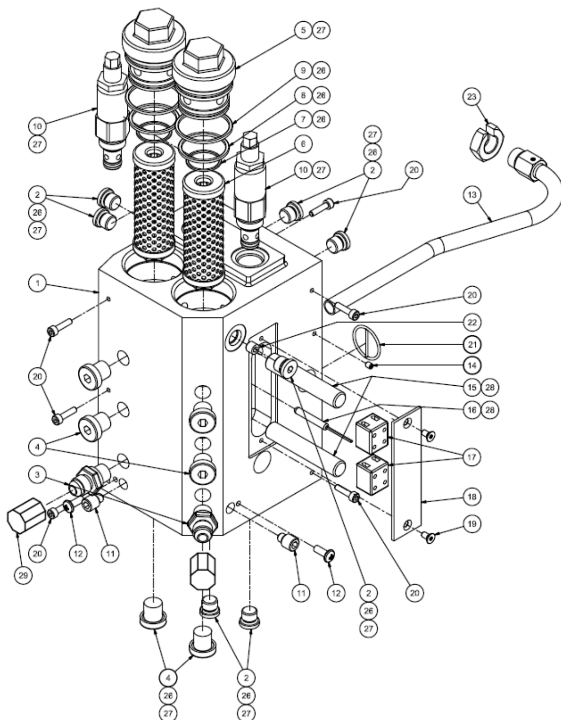
Illustration: Ensemble Collecteur de filtre à double sortie, SR5/10
