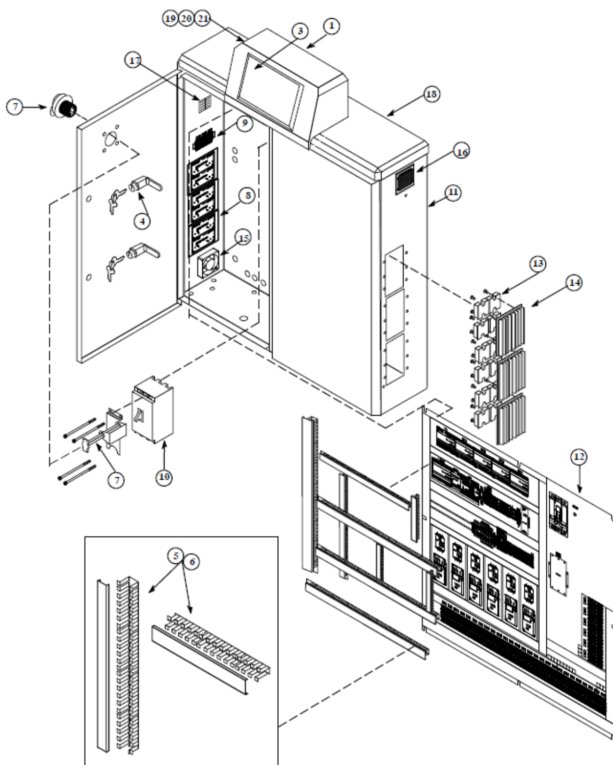
Darstellung: Typische Elektrischer Schaltschrank Baugruppe, M210 DCL V6
