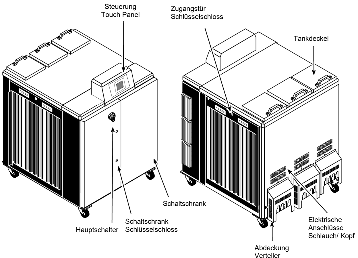
DYNAMELT M210 DCL Schmelzgerät
