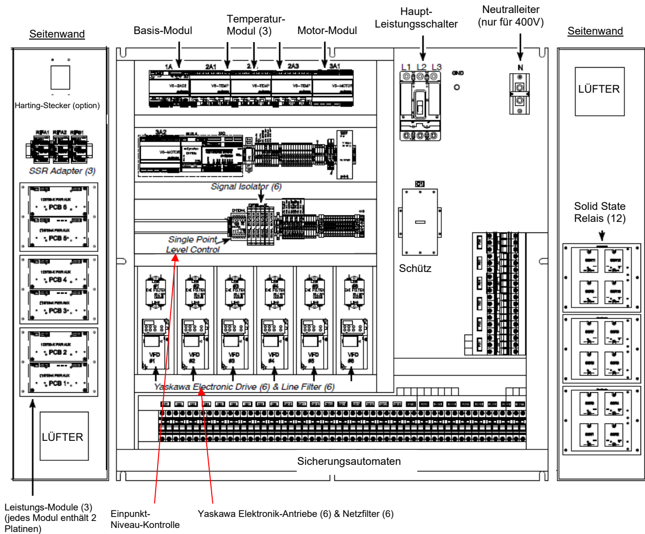
Typische Schaltschrank-Komponenten (Ein-Tank-Modell dargestellt)
