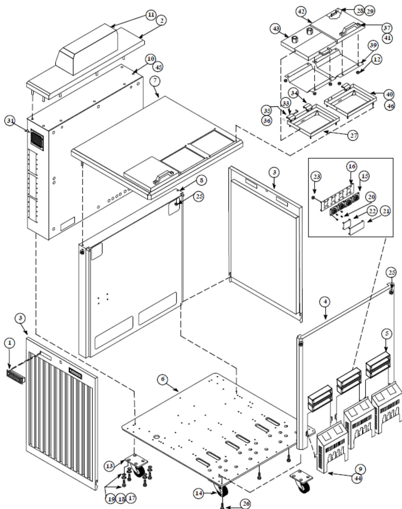
Darstellung: Schaltschrank Baugruppe M210, Art. Nr. 106047
