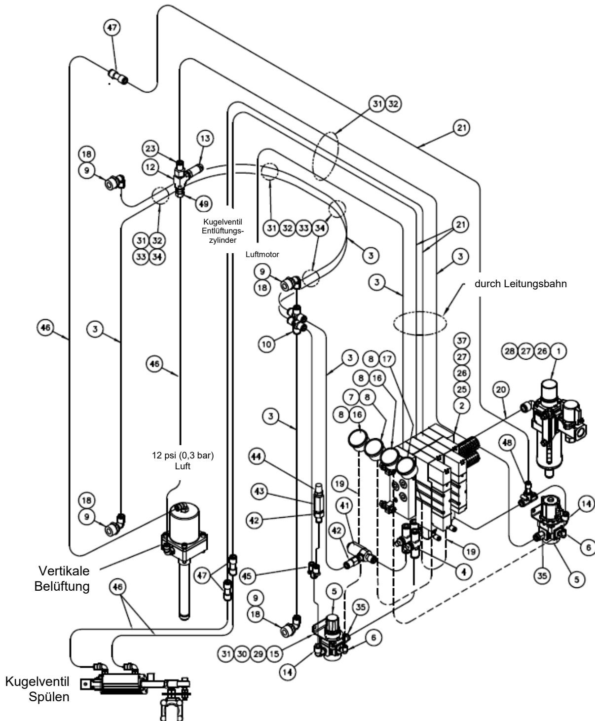
Abbildung: Pneumatikbaugruppe, DM55 PP, 5 PSI (0,3 bar) Vertikale Belüftung, Art. Nr. 823442
