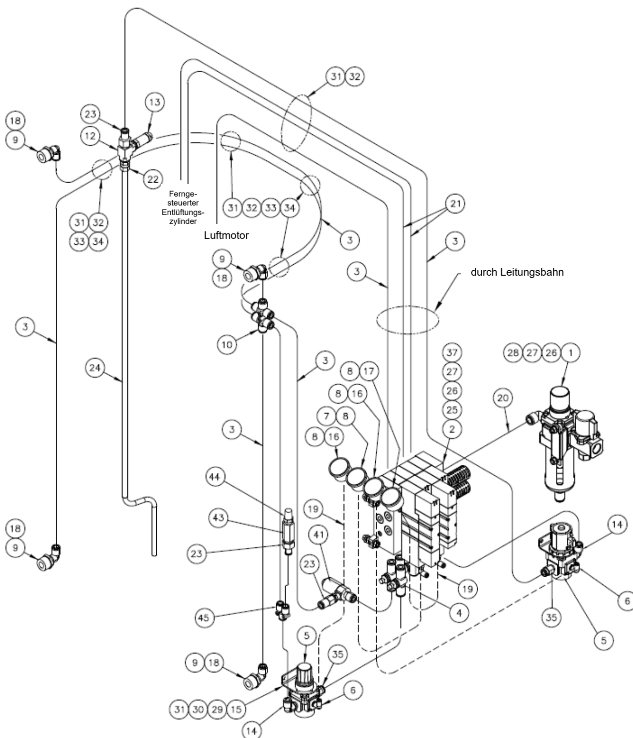
Abbildung: Pneumatikbaugruppe, DM55 PP, 5 PSI (0,3 bar) Belüftung, Art. Nr. 823064
