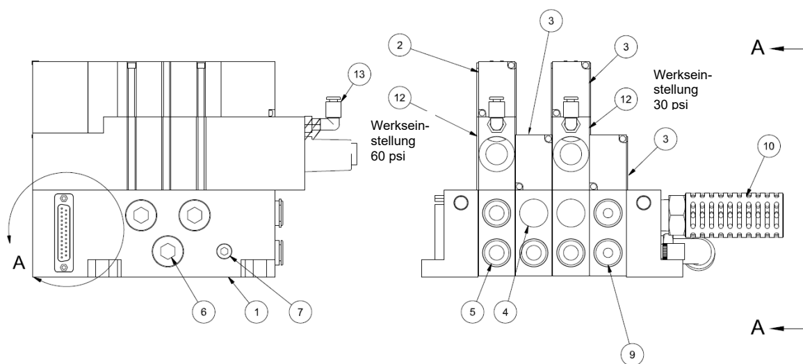
Abbildung: Ventilbaugruppe Kolbenpumpe, Art. Nr. 823066
