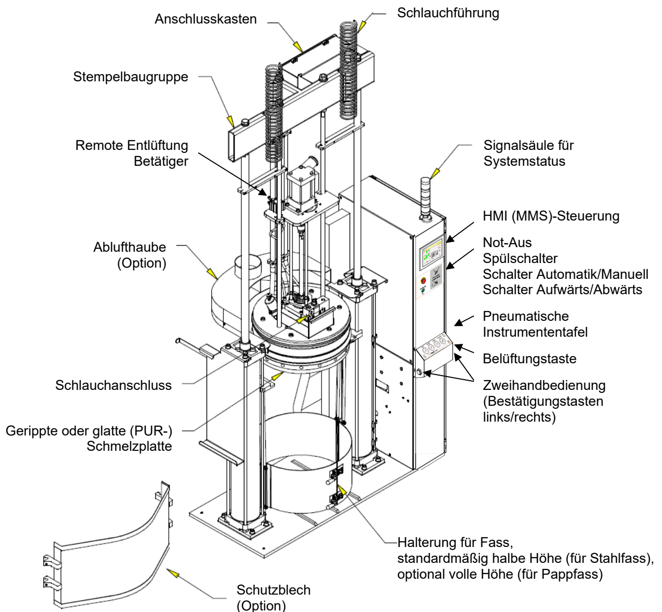
Abbildung: DM55 mit Kolbenpumpenkomponenten
