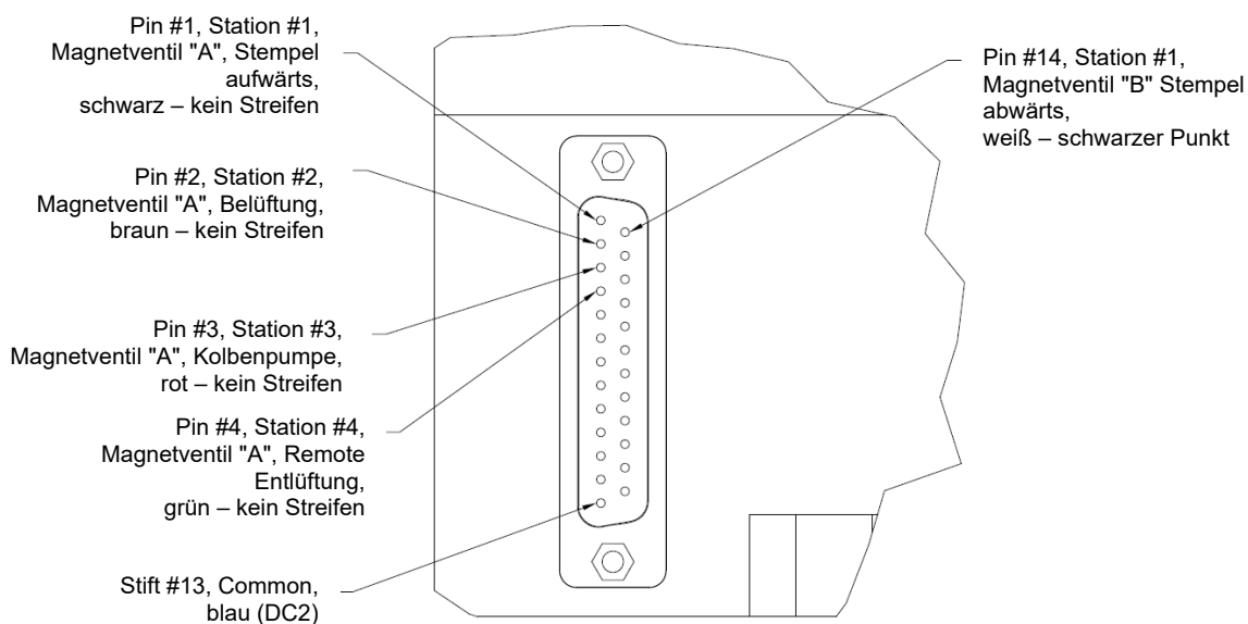
Pin-Bestückung Verbinder
