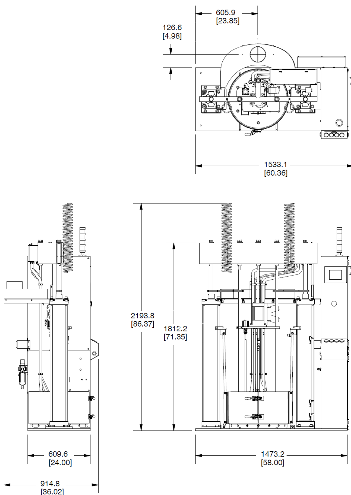
Installationsabmessungen des Fassschmelzers
