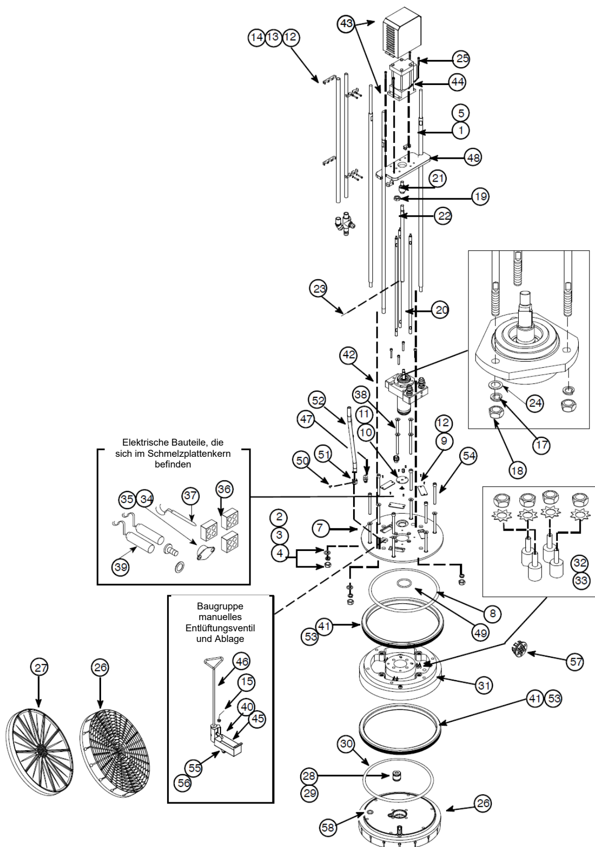
Abbildung: Baugruppe Heizstempel und Anschluss-Kit
